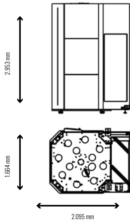
Beispiel: Abmessungen für die Baugröße M
