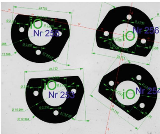
Mehr-Teile-Messungen für mehrere identische Teile auf einmal (MMi = Multiple Messung identisch).
